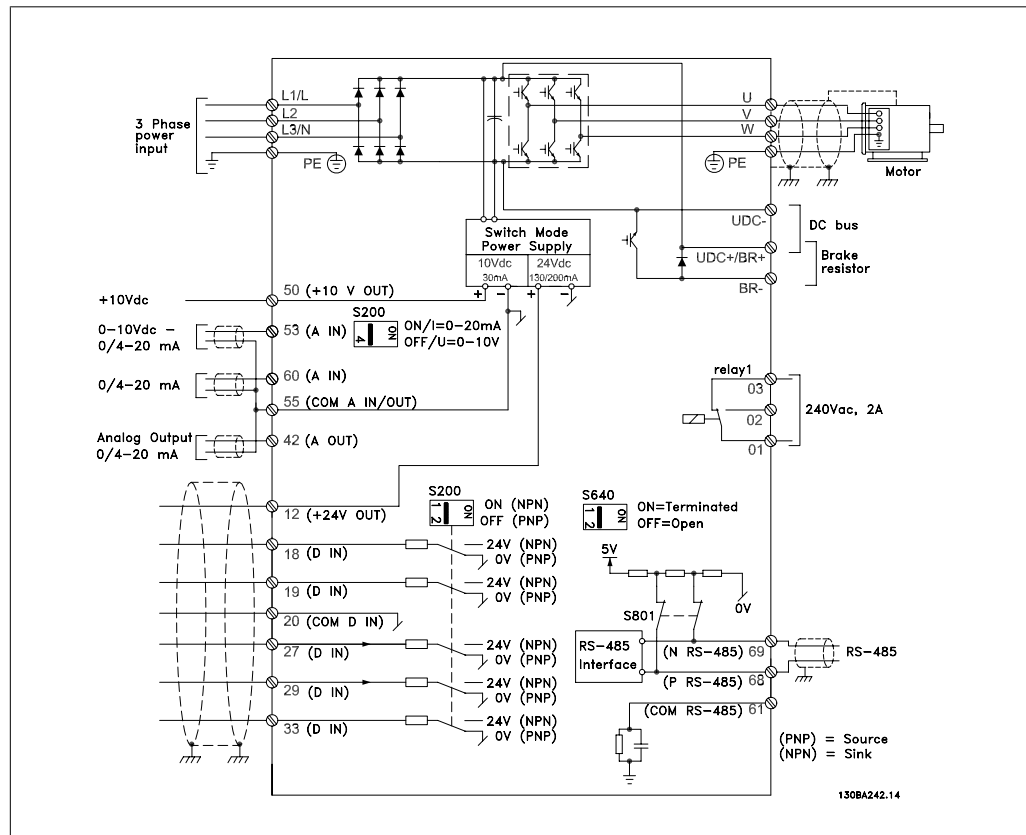
Çizim 3.10: Tüm elektrik terminallerini gösteren diyagram.
