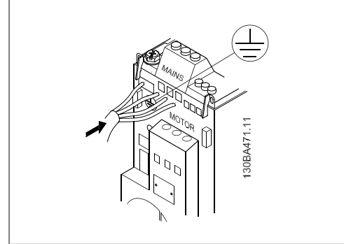
Çizim 3.1: Toprak kablosunun ve şebeke tellerinin montajı.
